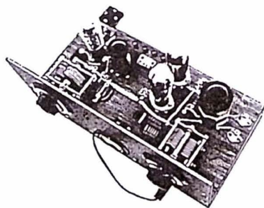
Fig. 12 - Trasmettitore radiotelegrafico del 1934 costituito da un oscillatore a cristallo con tetredo tipo "47" ed amplificatore A.F. con due tetredi tipo "46" in parallelo, impiegati come triodi. Con la tensione di placca di 500 V, la potenza ingresso poteva essere di 50 W.
